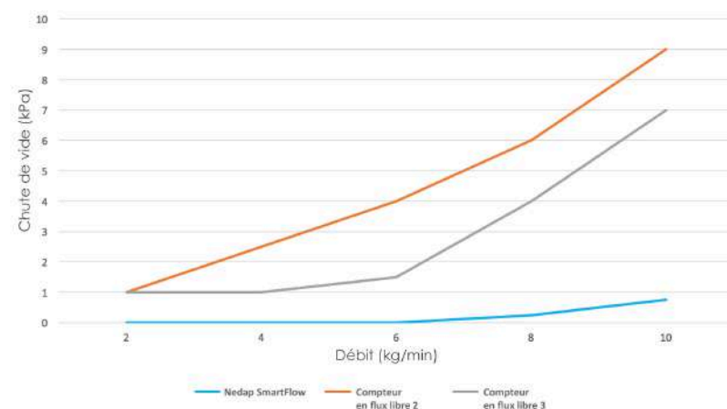
Chute de vide concernant le débit du Nedap SmartFlow par rapport à deux compteurs à lait en flux libre classiques. ▲
