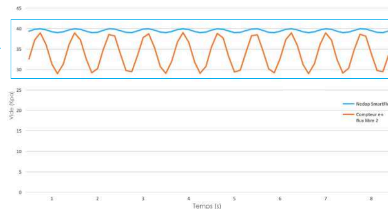
Fluctuations de vide à un débit de 6 kg/min du Nedap SmartFlow par rapport à un compteur à lait en flux libre classique. ▲
